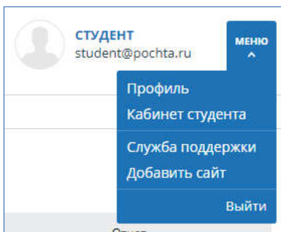
Рисунок 4. Выпадающее меню
